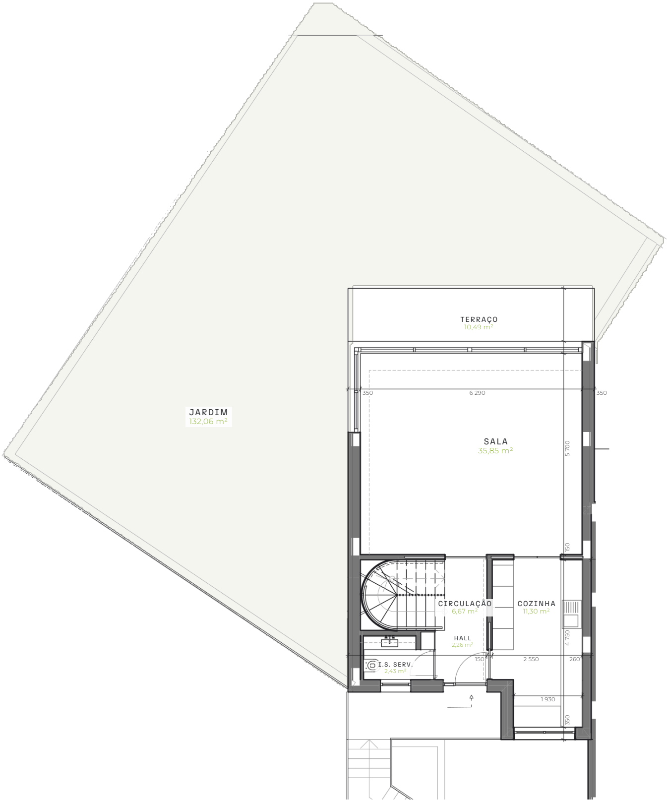
RÉS-DO-CHÃO
