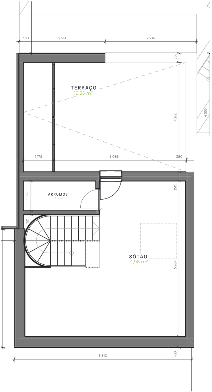
SÓTÃO ATTIC · 43,46 M²
